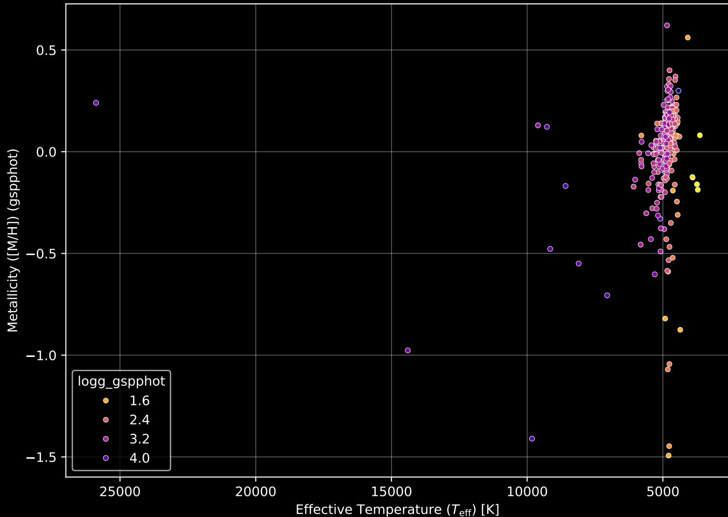
APOGEE DR17 Field: [326+06] Stellar Population Parameters (n= 277)
